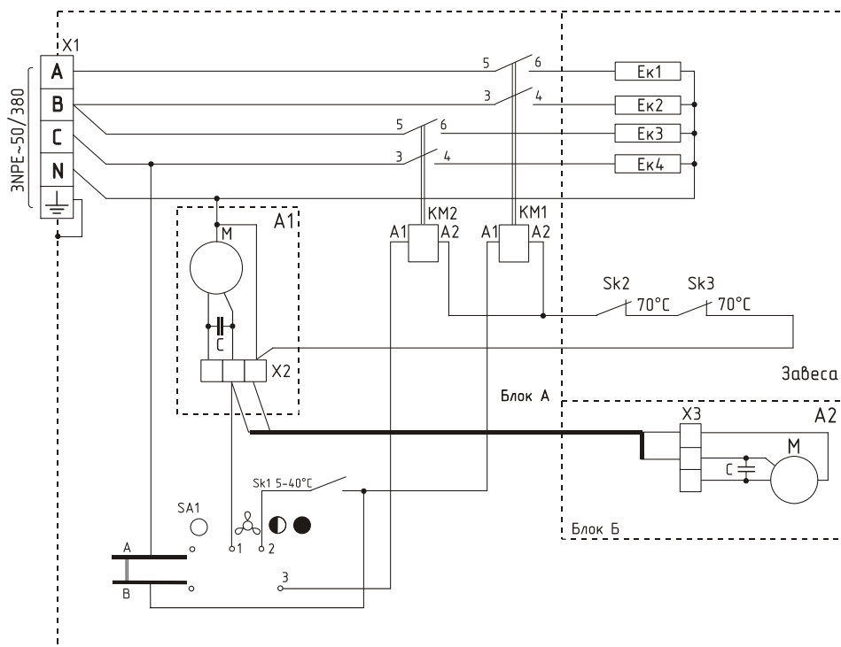
Рис. 10 Электрическая схема завес КЭВ-8П1060Е, КЭВ-10П1060Е
